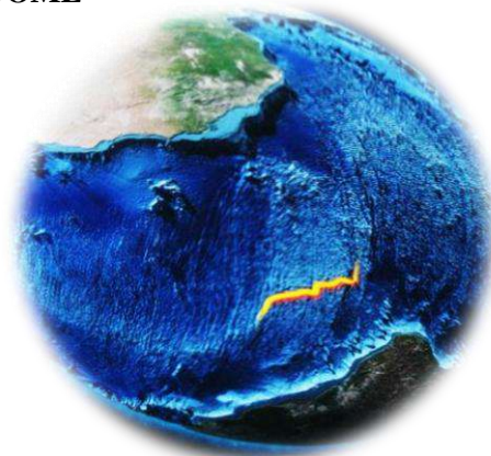
Proiecție – Imaginea unei falii tectonice pe Terra, luată din spațiu
